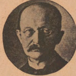
MAX PLANCK
