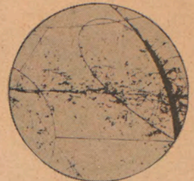
NEUTRINO
