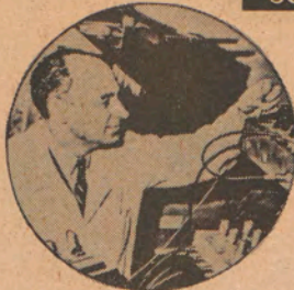
ENRICO FERMI
